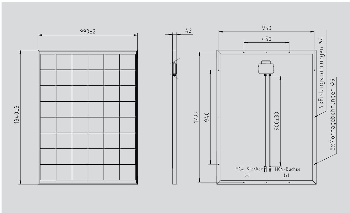
Maßzeichnung IBC PolySol 180 GE
