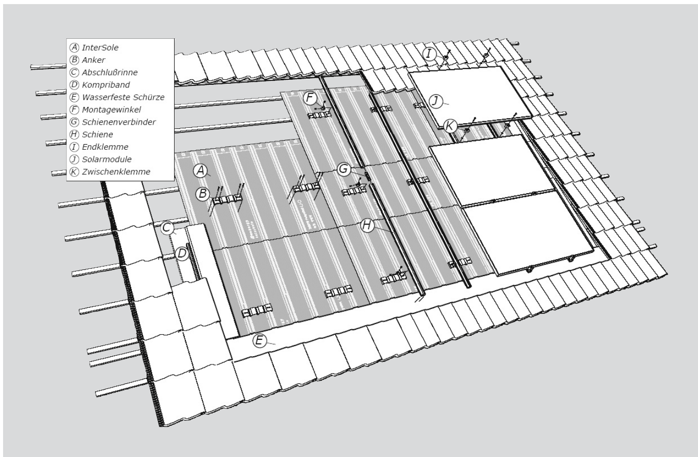
Montageschema
